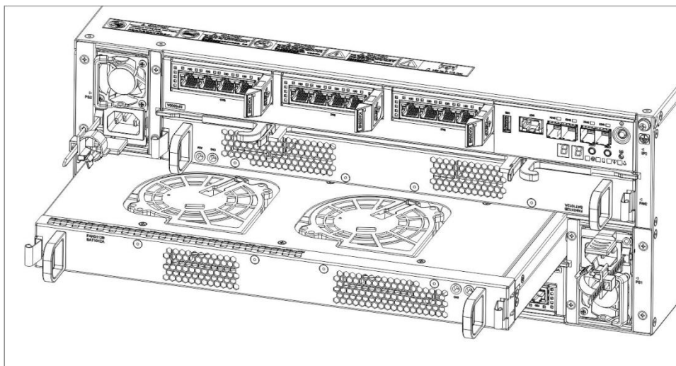
图6-2 安装/拆卸 SPU 风扇模块+电池模块示意图
