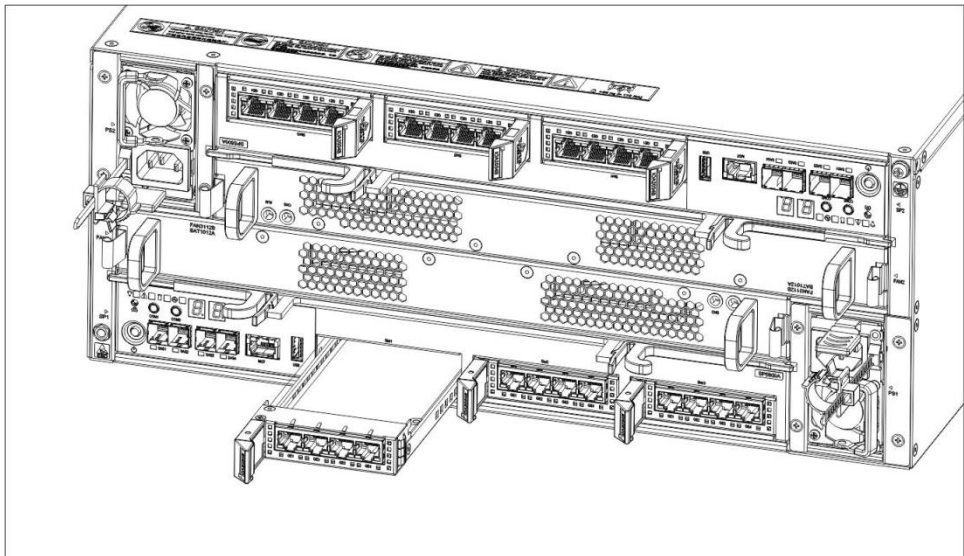
图6-4 安装/拆卸 IO 插卡示意图
