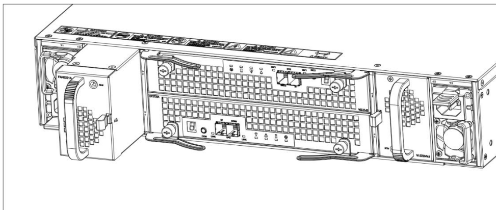
图6-10 安装/拆卸 DSU2725 后端风扇模块示意图
