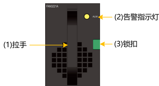
图3-20 DSU2725 后端风扇模块正视图
