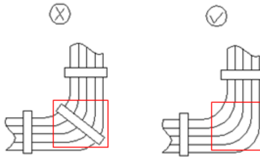
图4-20 线缆捆扎示意图（三）
