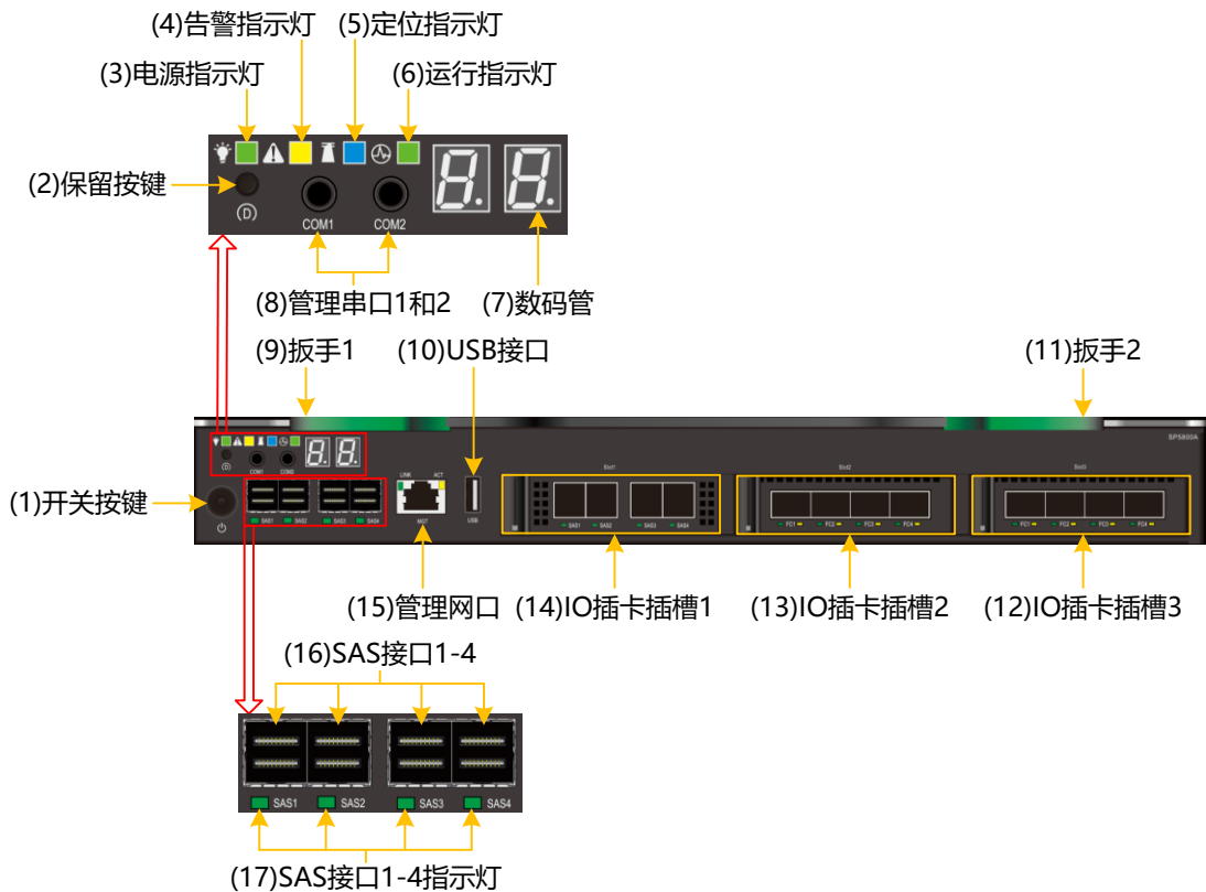
图3-3 SP 正视图
