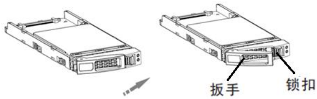
图6-16 安装 2.5 英寸磁盘模块 A 示意图（一）
