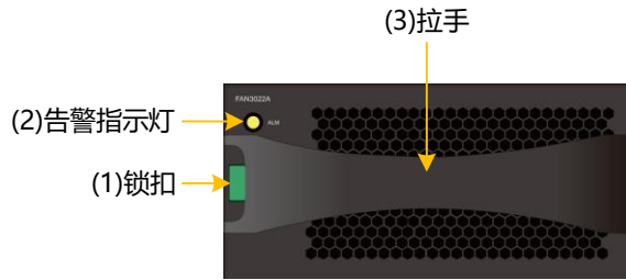
图3-15 DSU2624 风扇模块正视图
