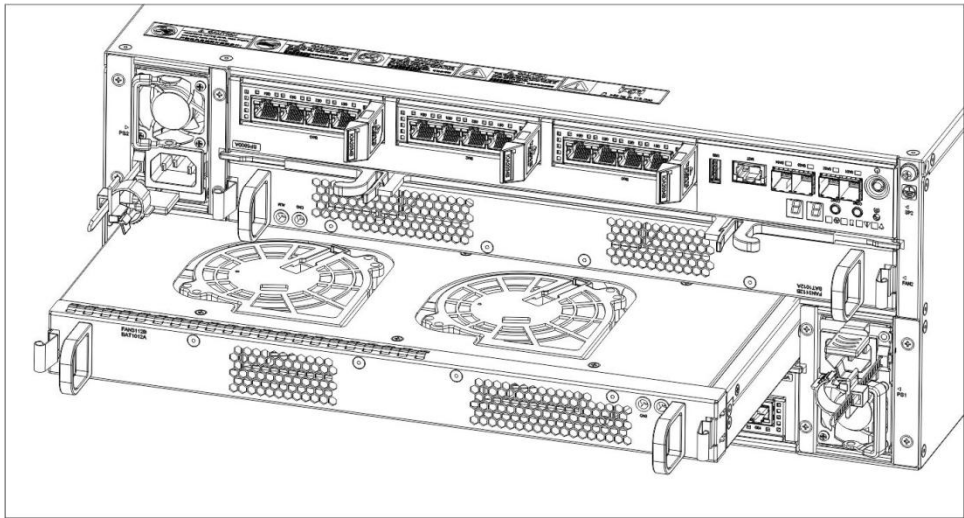
图4-14 安装/拆卸 SPU 风扇模块+电池模块示意图
