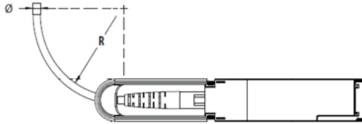
图4-32 AOC 光缆弯曲半径示意图
