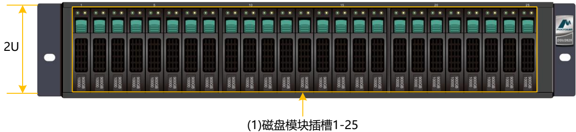
图3-7 DSU2625 前正视图
