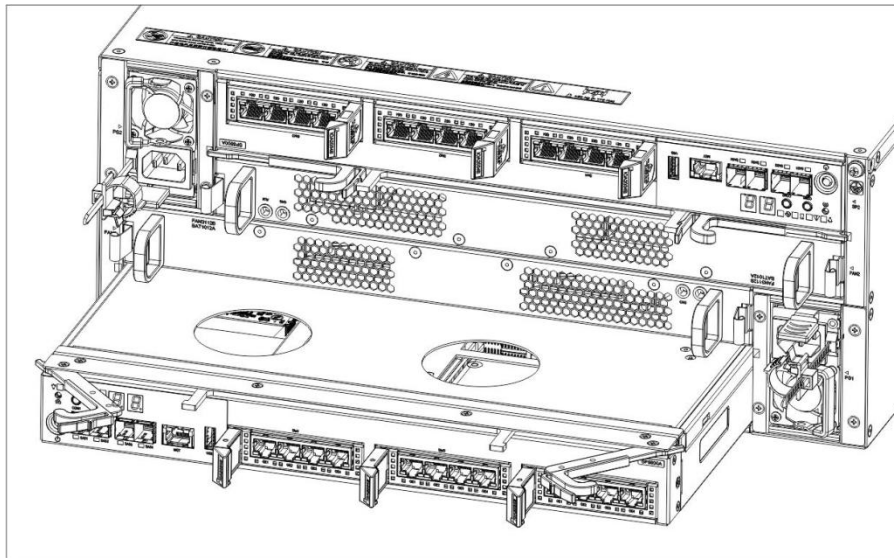
图6-1 安装/拆卸 SP 示意图
