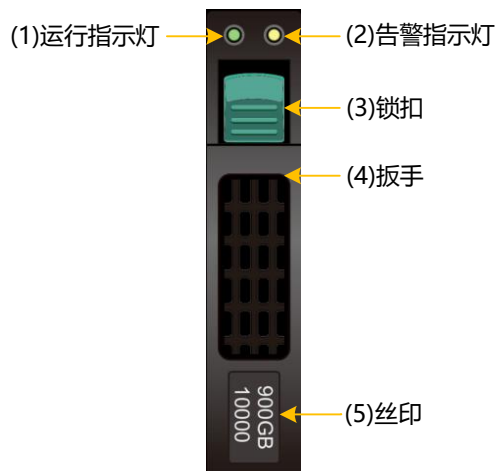
图3-26 2.5 英寸磁盘模块前面板
