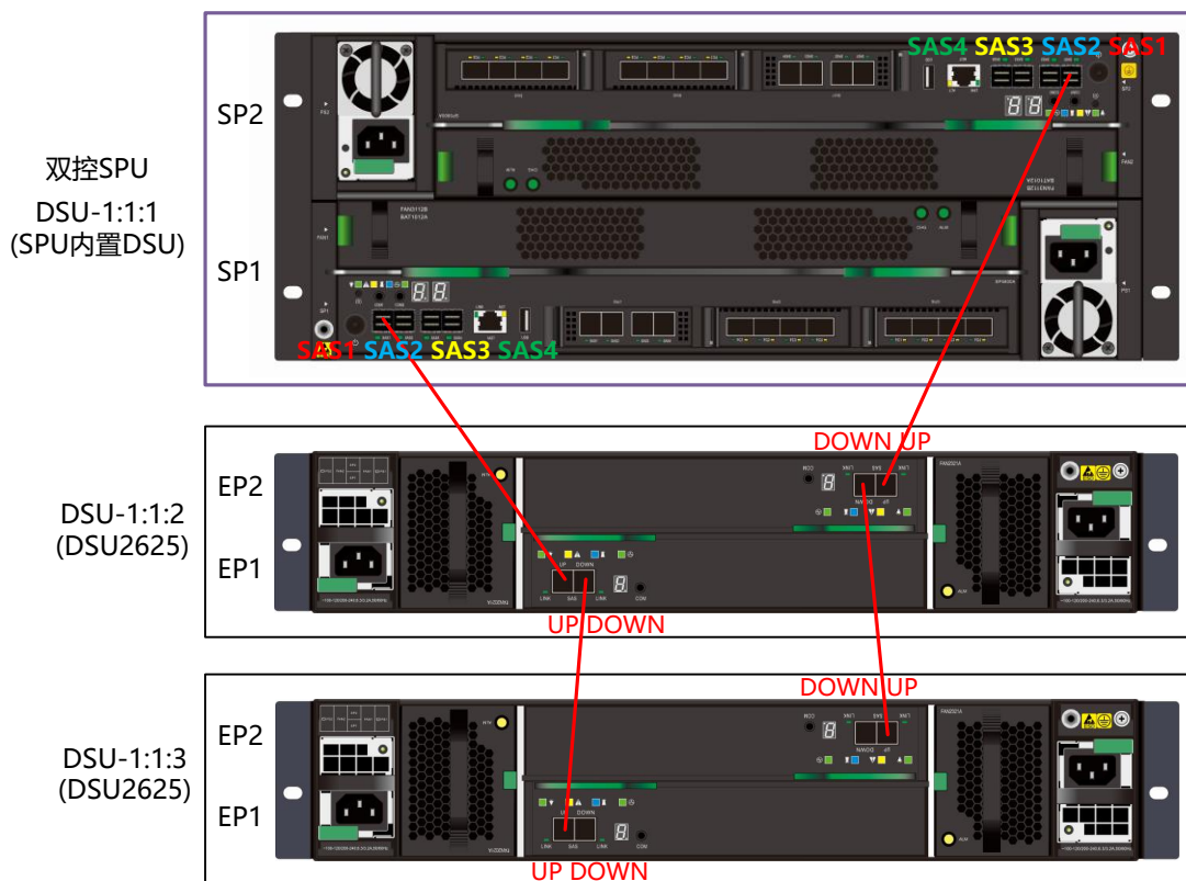
图4-33 SAS 线缆安装示意图
